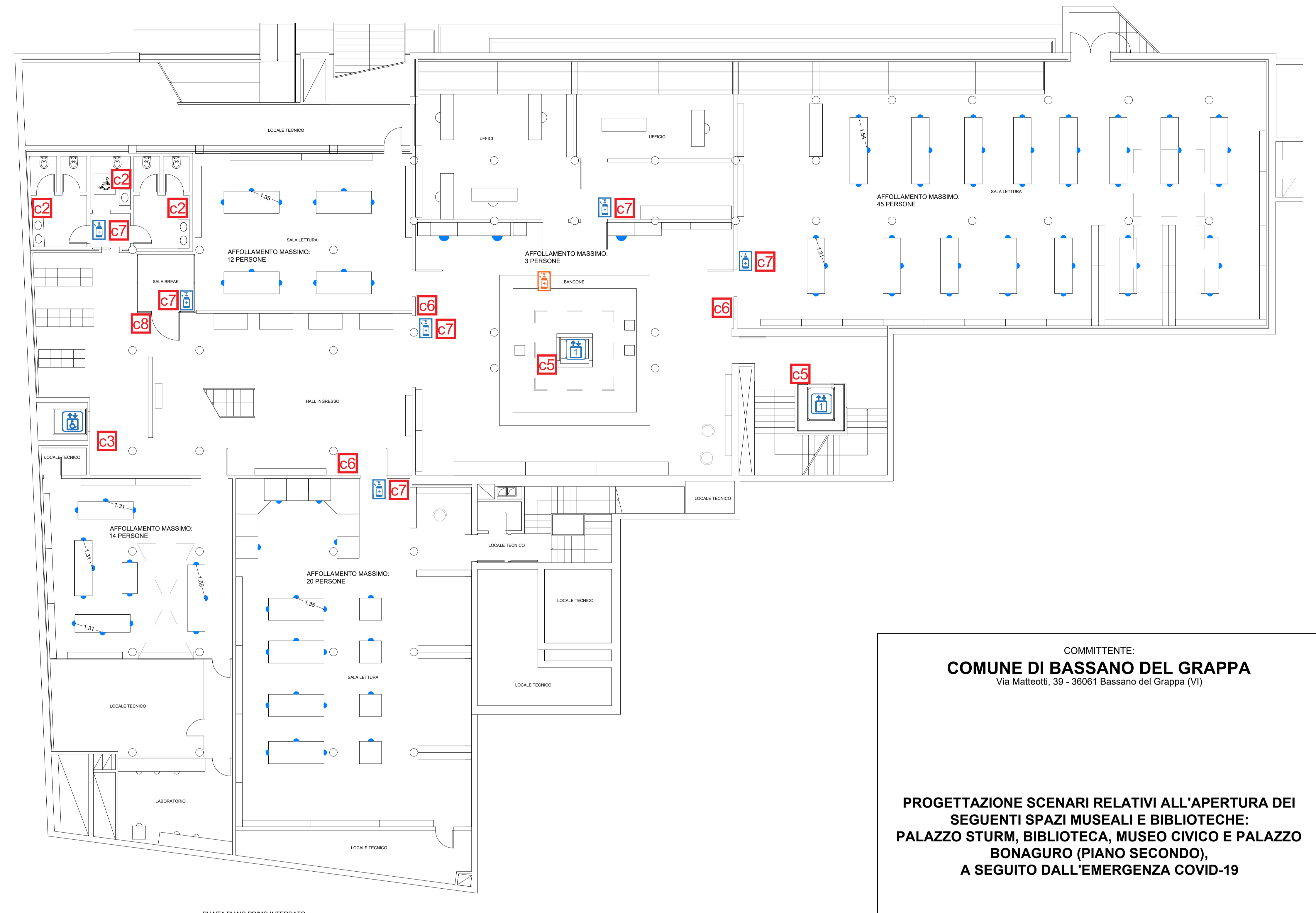
PIANTA PIANO PRIMO INTERRATO
